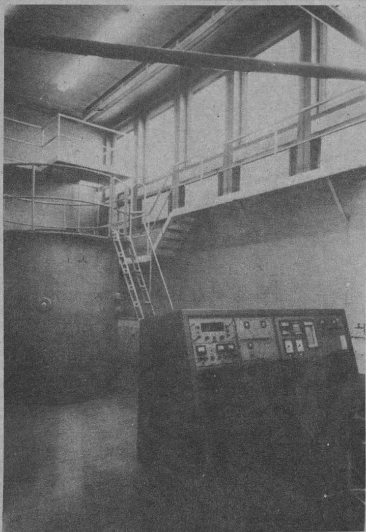
Un aspecto de la consola y del reactor donado a la UNAM para la enseñanza y la investigación científicas. Quedará instalado en el recinto del Laboratorio Nuclear, frente al edificio del Centro de Investigación de Materiales.
